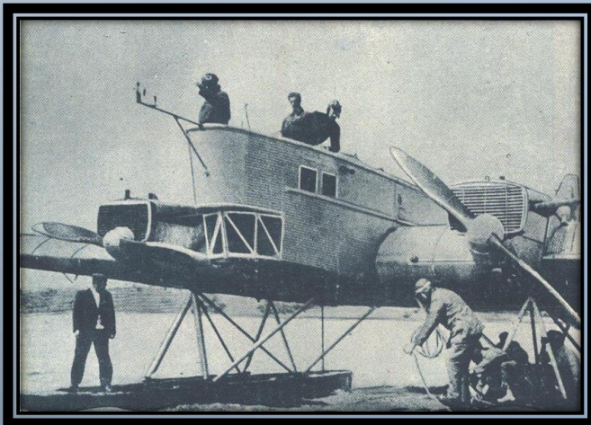
Серийный экземпляр ТБ-1 (АНТ-4)
